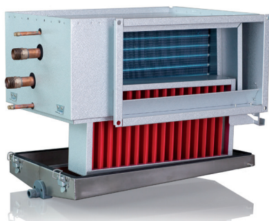
PGK z zamontowanym separatorzem wody, DE
