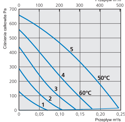
CIŚNIENIE/PRZEPŁYW F7-filter Przepływ m 3 /h
